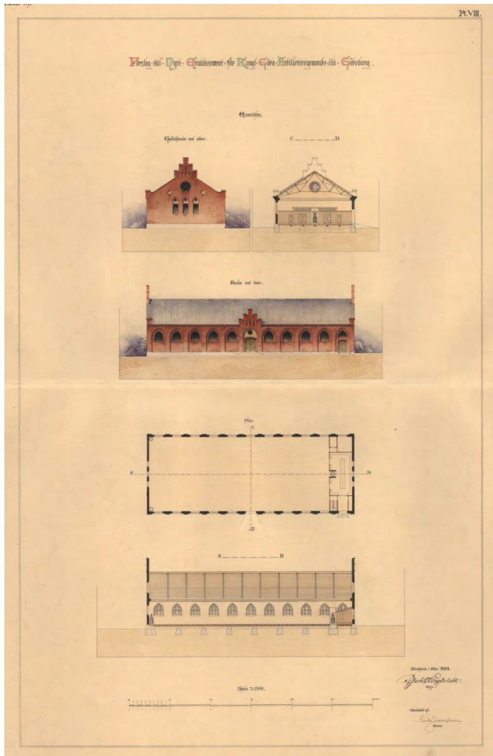
Originalritning av exercishuset från 1891 av Erik Josephson. (Krigsarkivet)
