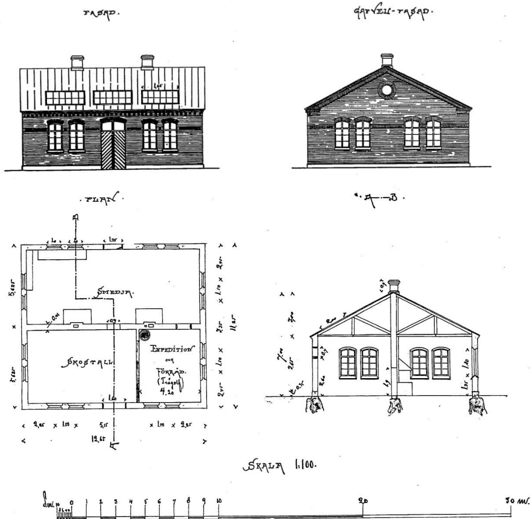
Ritning över skostallet, okänt årtal. (Kaas, 1998)
