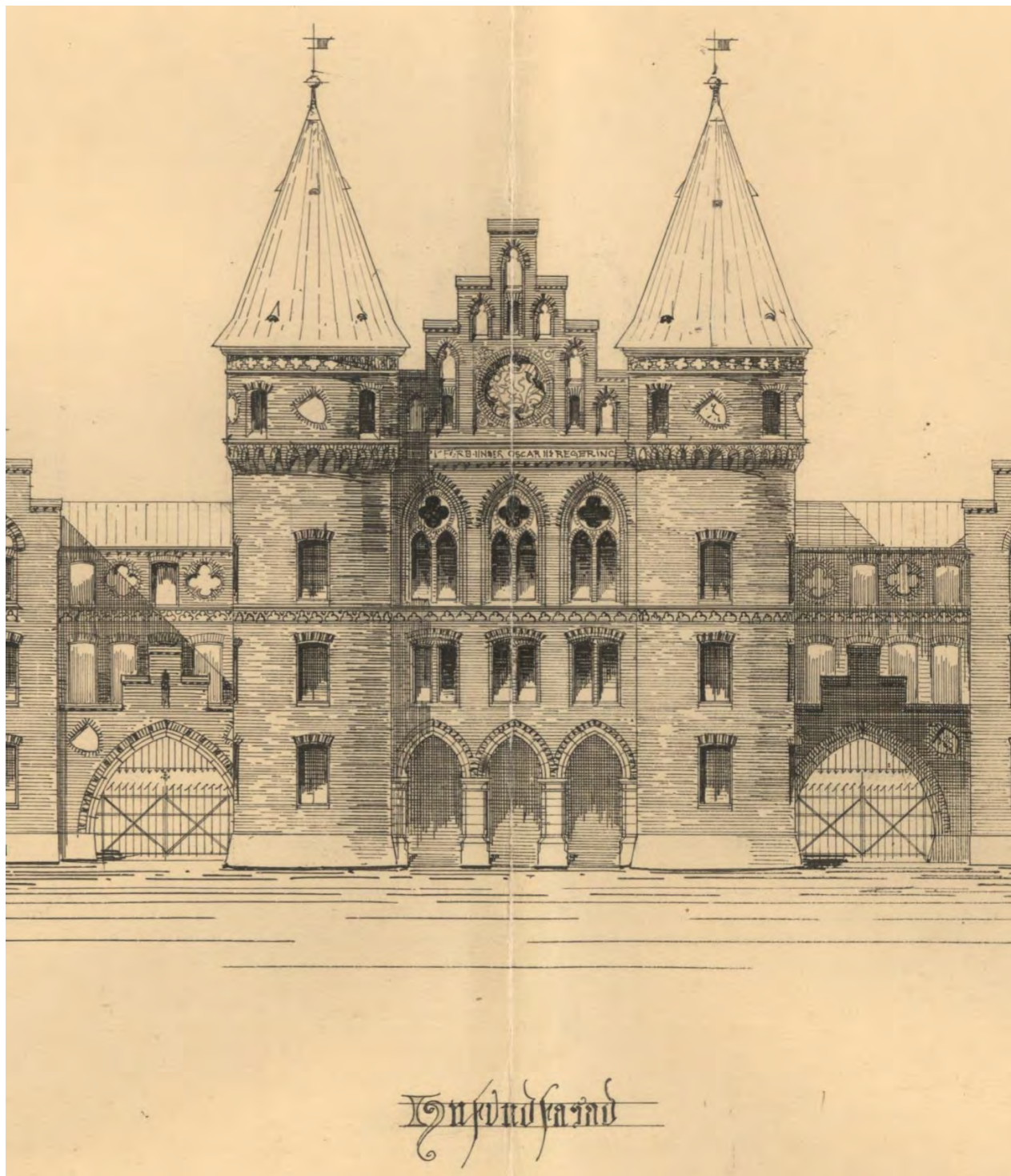
Originalritning av kanslihuset från 1891 av Erik Josephson. Detalj, södra fasaden. (Krigsarkivet)
