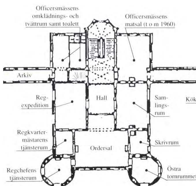
Planritningar över kanslibyggnaden. (Kvibergs kaserner, 1994)
