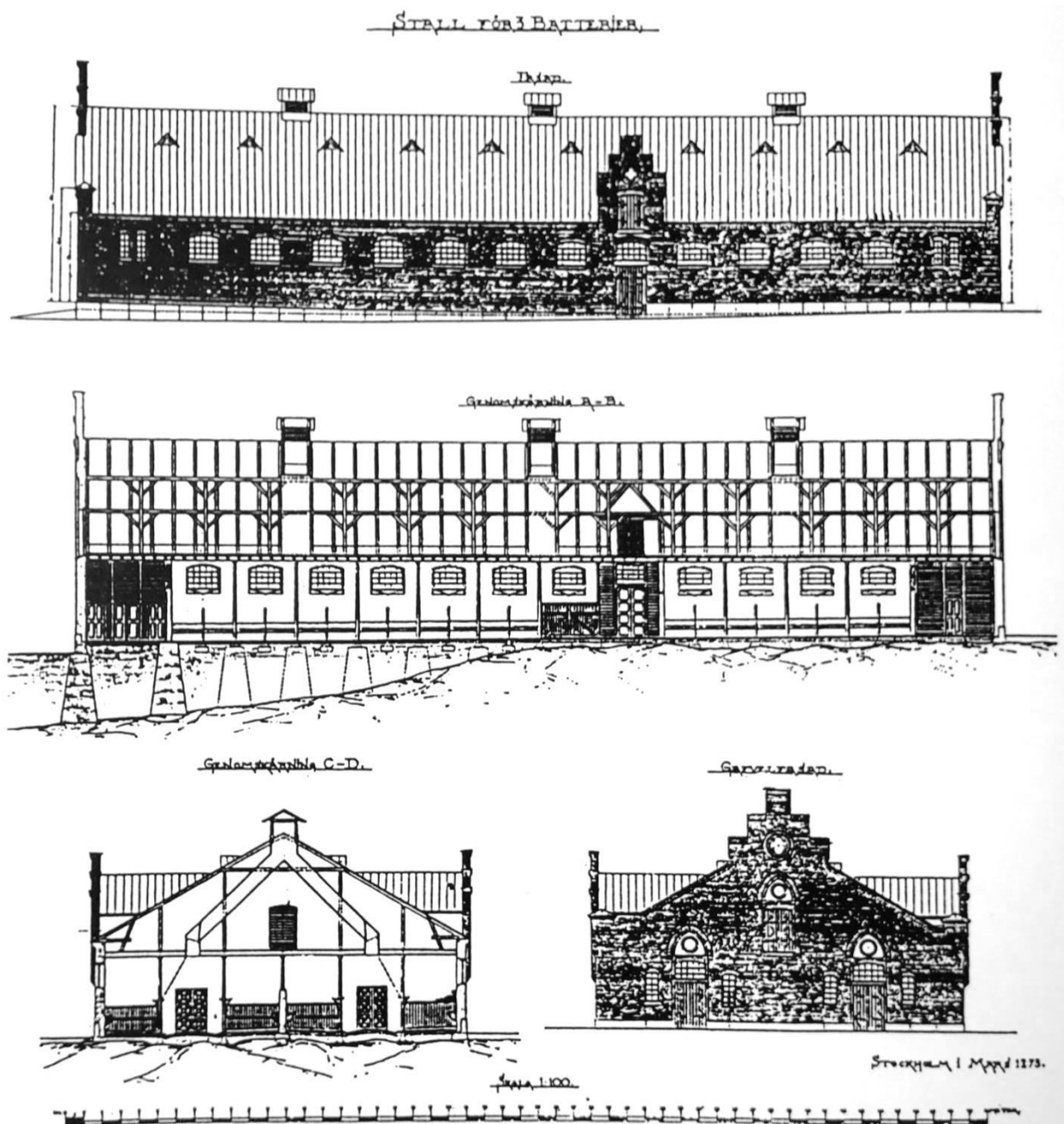
Originalritning av stallbyggnaderna från 1893 av Erik Josephson. (Kvibergs kaserner, 1994).
